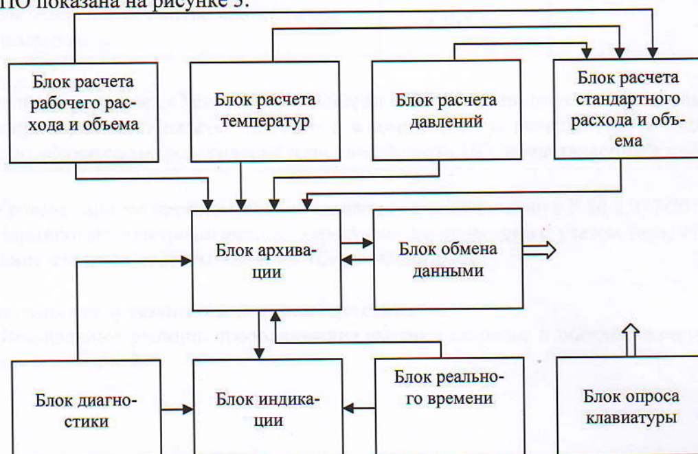
Рисунок 3 - Структура ПО
